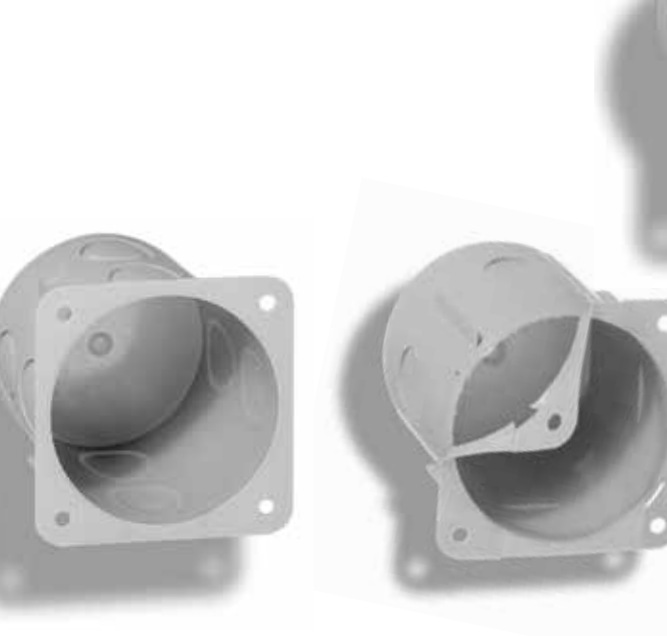
HSB Boîtes pour constructions légères FID 850° 2x1, 50 mm No E 372 604 676
