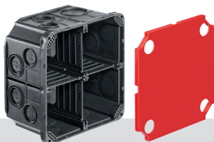
HSB Einlasskasten Vario
