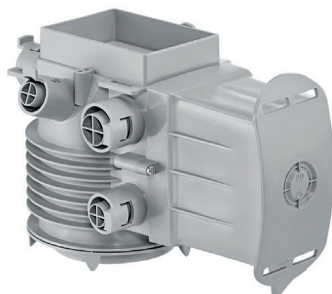
EB-Gehäuse Tunnel 90 mm
